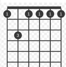
Fmi
