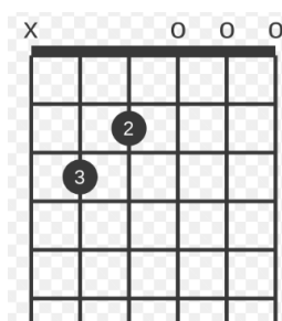
Cmaj7
